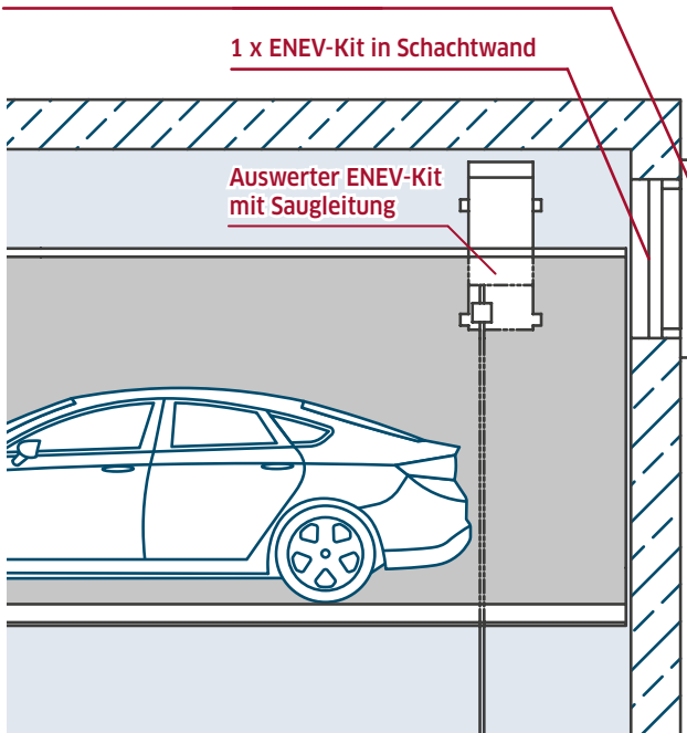
Schematische Darstellung Wetterschutzabdeckung bauseits
