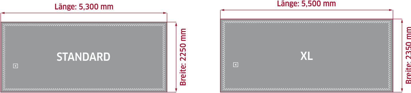
Abb.5: Palettengrössen im E-PUZZLE® System.
