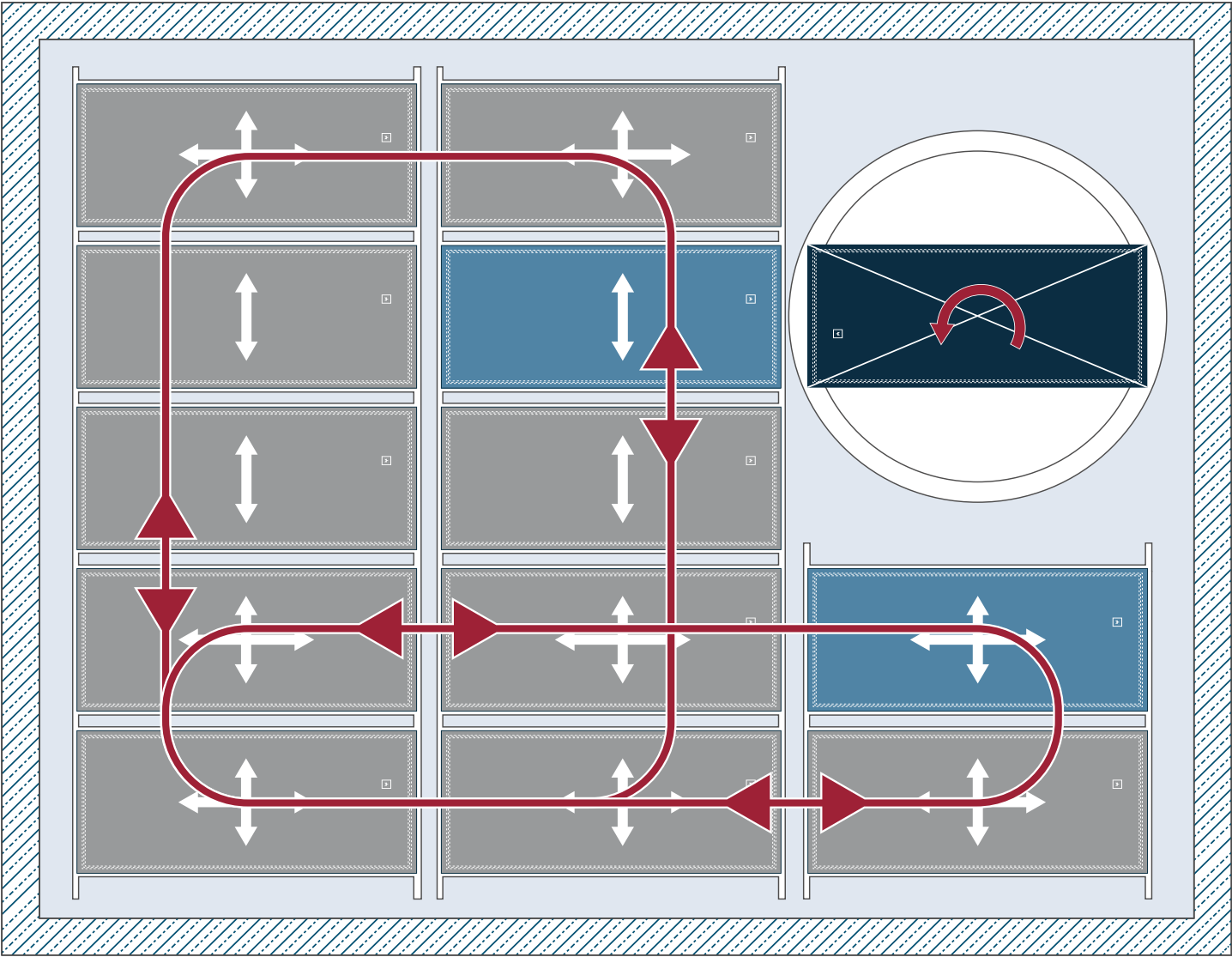
Abb.10: Drehtisch in Parkebene.
