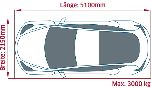
Abb. 3: Fahrzeugmasse für das Parksystem E-PUZZLE®.
