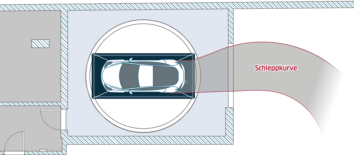
Abb.11: Drehtisch in Kabine.
