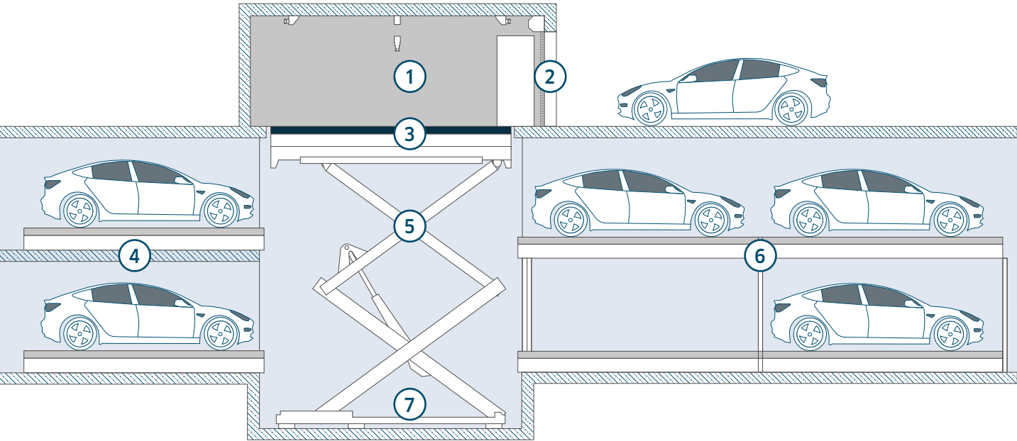
Abb. 4: Das Parksystem E-PUZZLE®.
