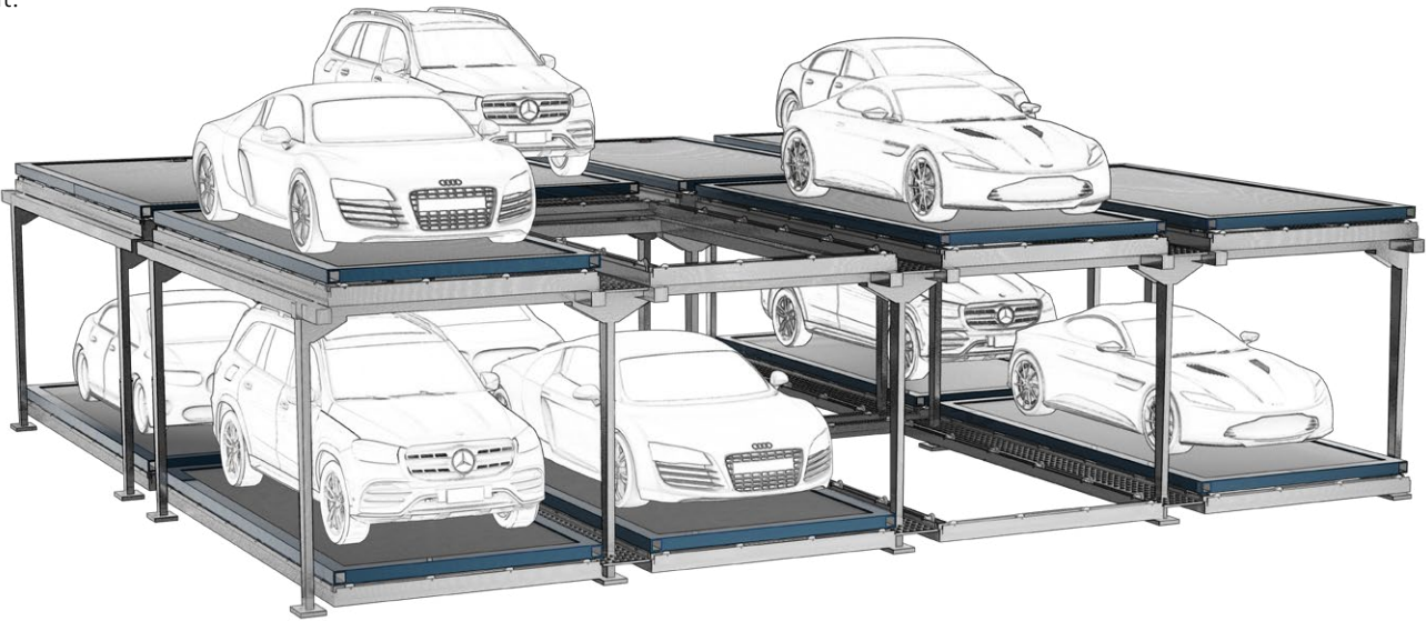
Abb. 2: 3D Abbildung des E-PUZZLE® Parksystems mit 12 Stellplätzen in Stahlbauweise.
