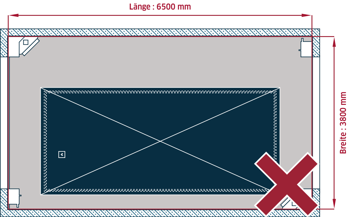
Abb. 17: Inkorrekte Platzierung des Hebers in der Kabine, da sich die Palette nicht mehr in einer Flucht mit dem Kabinentor befindet..
