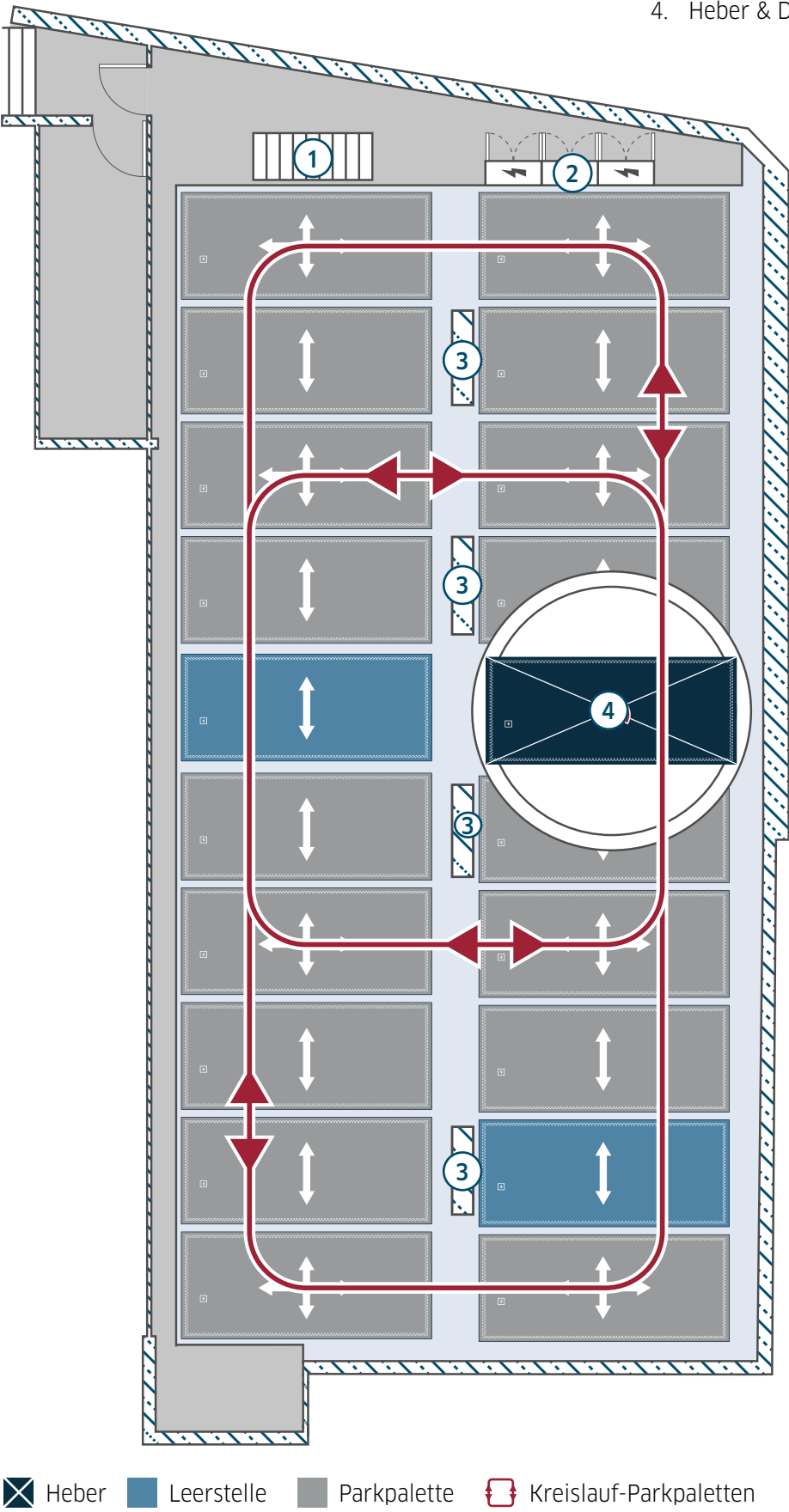
Abb.21: Komplette Systemübersicht E-PUZZLE® mit Zugängen, Schaltschränken und Wartungszugängen.
