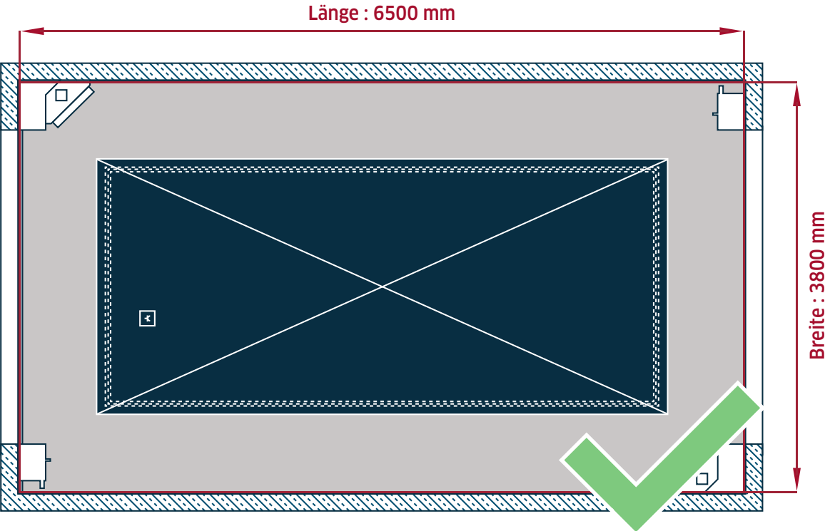
Abb. 16: Korrekte Platzierung des Hebers in der Kabine.
