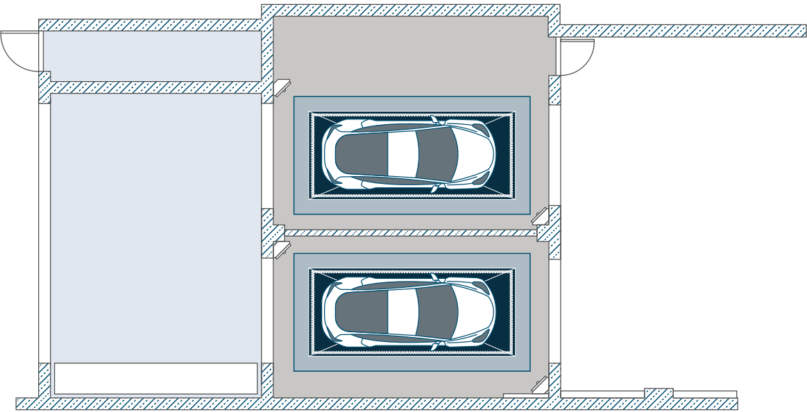
Abb.15: Draufsicht einer Doppelkabine.
